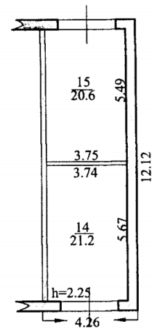
Поэтажный план помещения в здании гражданского и производственного назначения М 1:200
